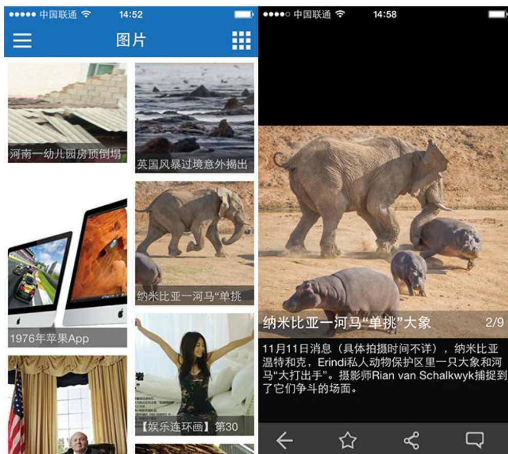
图 17 组图展示
