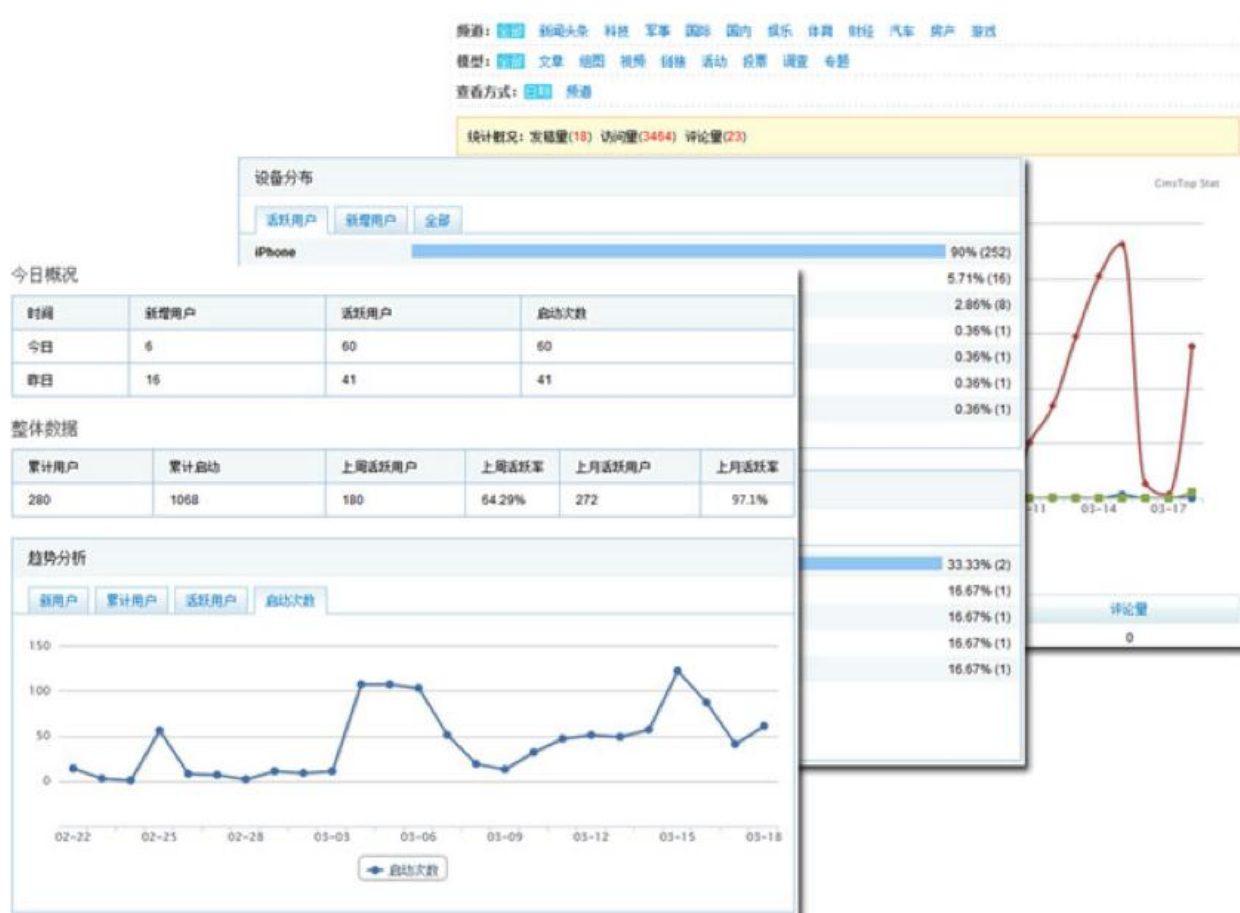
图 29 图表统计
