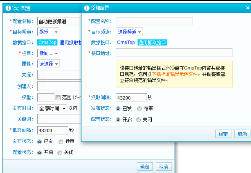
图 40 添加配置
