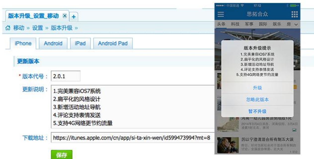
图 43 版本升级
