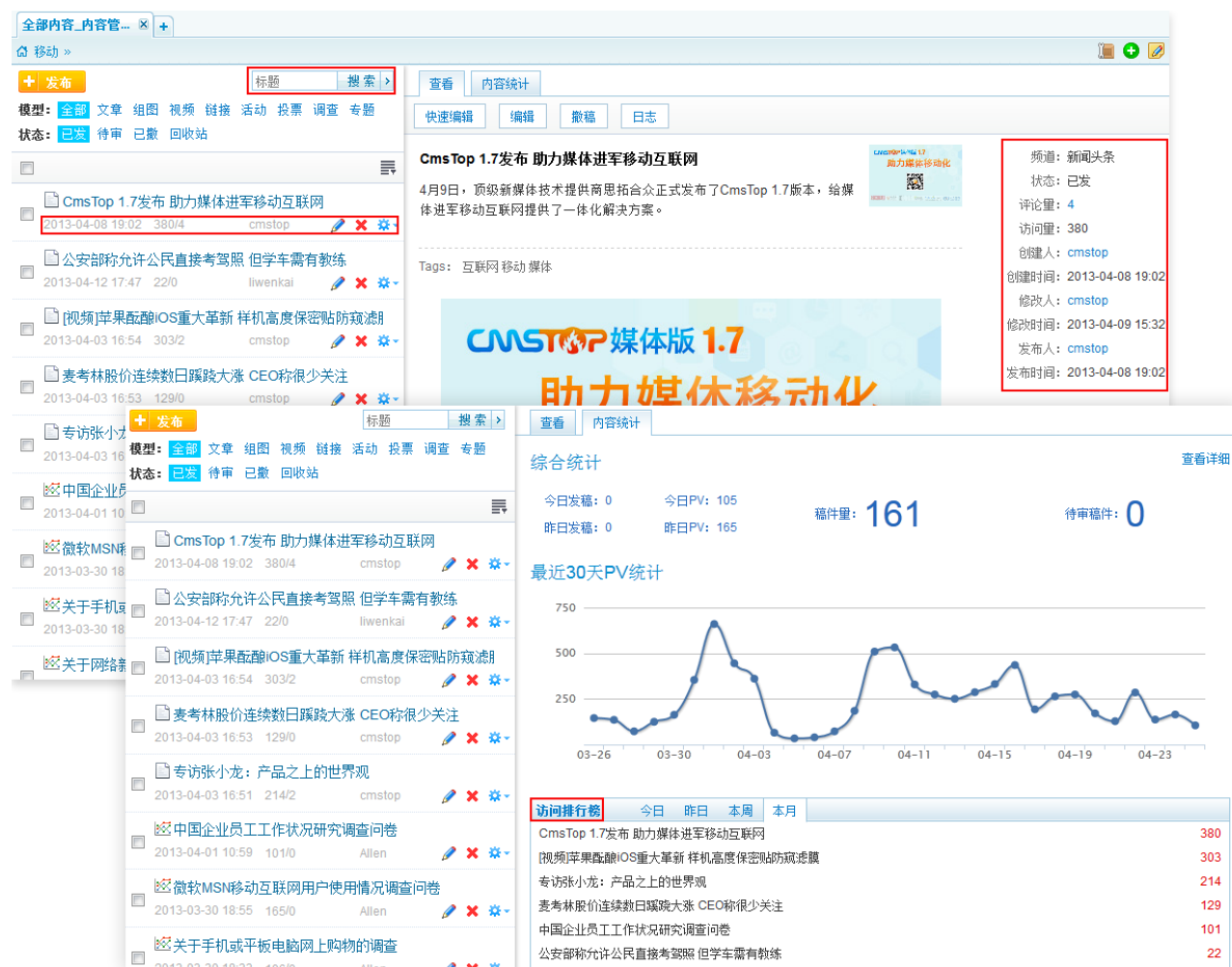
图 23 后台界面
