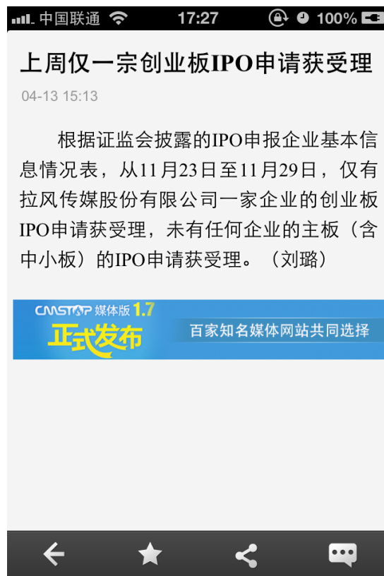
图 32 内容页广告
