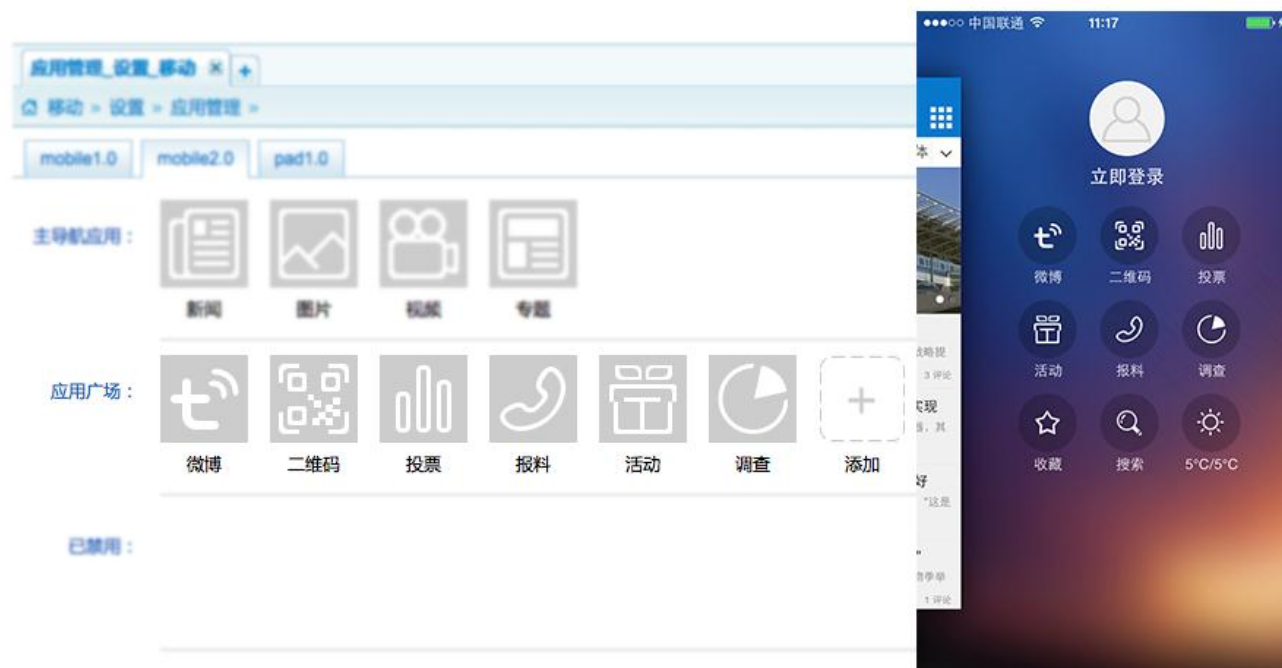
图 41 应用管理
