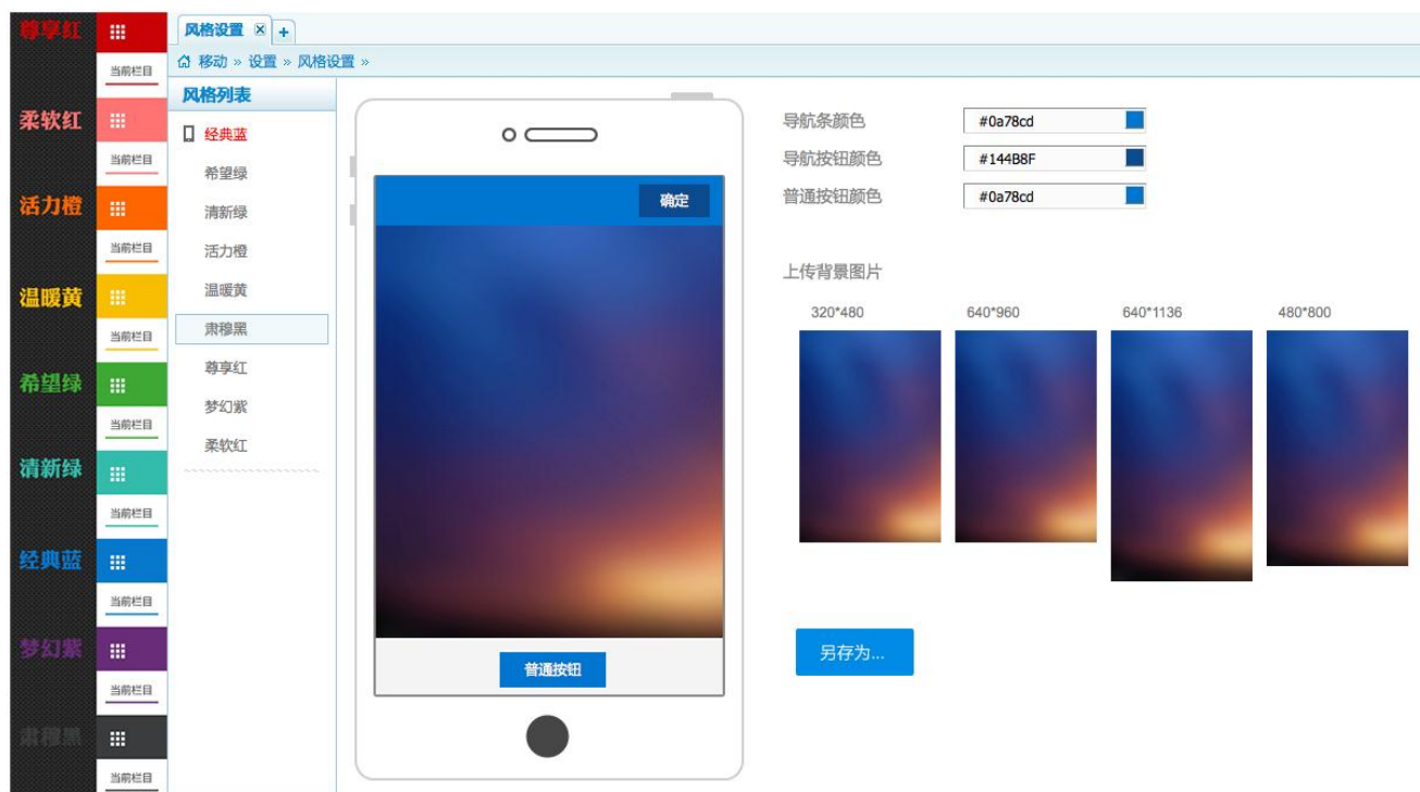
图 45 多套皮肤
